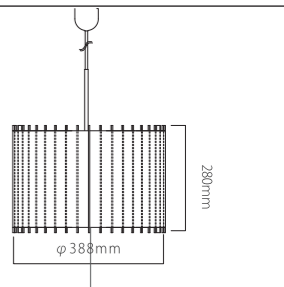
ST-P 全体サイズ(コード長含む): H800mm×Φ388mm シェードサイズ: H280mm×φ388mm ランプ: 100W ボール球 2灯式ペンダント (100W×2, 切り替えスイッチ付/2灯→1灯→ナツメ球) 色種類: 機械漉き和紙(白)・民芸紙(黒・赤・紫)
